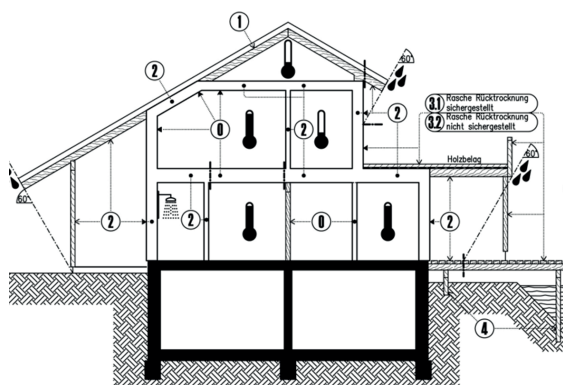
Figura 4.1) ÖNORM B 3802-1 – Locali e classificazioni delle classi d'uso in funzione delle condizioni di umidità dell'ambiente e se lo stesso è riscaldato o meno durante l'anno
