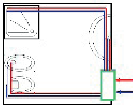
Figura 2.7) Distribuzione impianto idraulico senza accavallamenti e con collettore.
