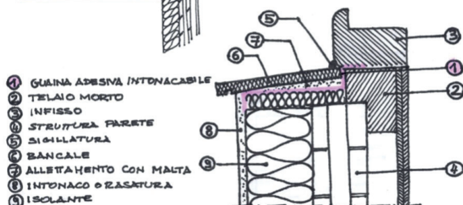
Figura 2.4) Sigillatura a forma di vasca con guaina adesiva preferibilmente butilica; la guaina deve essere risvoltata verso l'alto sotto la finestra contro il telaio morto e verso il basso e sui lati del cappotto a livello della facciata.
