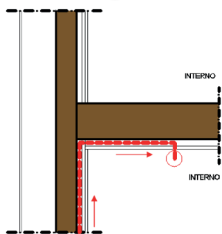
Figura 2.16: Passaggio corretto del punto luce.
