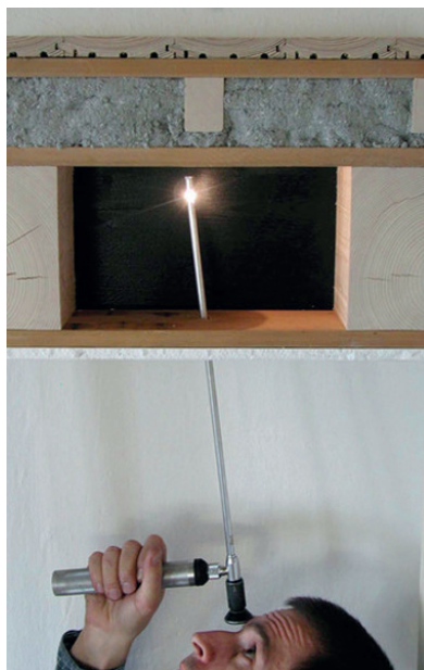
Figura 3.1) A sinistra: perforazione del pacchetto costruttivo; a destra: ispezione mediante endoscopio
