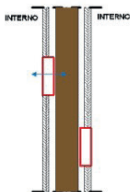
Figura 2.15: Posizione corretta delle scatole elettriche
