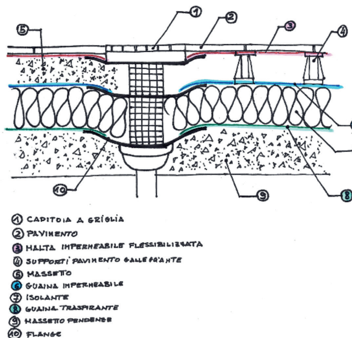
Figura 2.1: Esempio di capitoia con raccordi ai vari livelli di guaina
