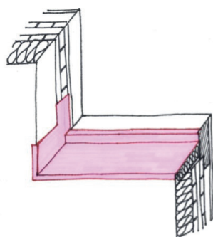
Figura 2.4) Sigillatura a forma di vasca con guaina adesiva preferibilmente butilica; la guaina deve essere risvoltata verso l'alto sotto la finestra contro il telaio morto e verso il basso e sui lati del cappotto a livello della facciata.
